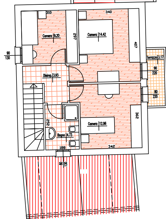
Piano primo
